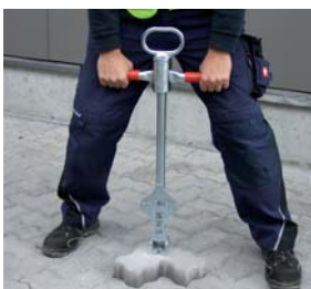
Przyrząd do wyciągania kostki SZH
